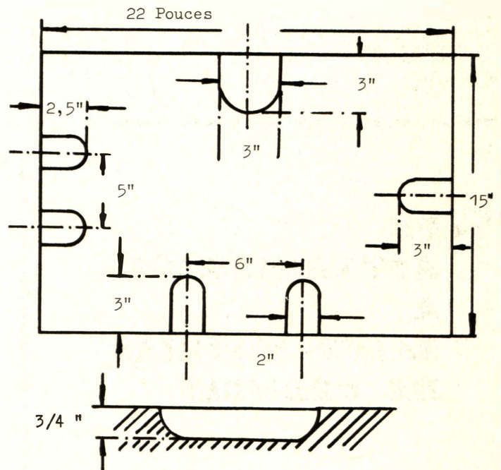
Dimensions d'un pied d'atterrissage
